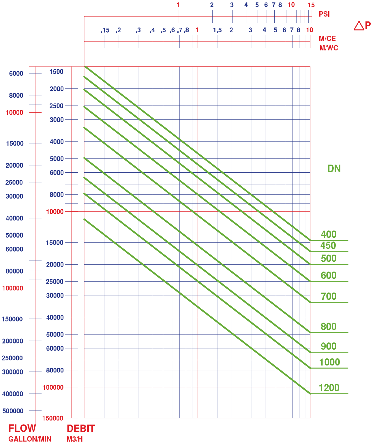
Diagramme de pertes de charge ( \Delta p )
